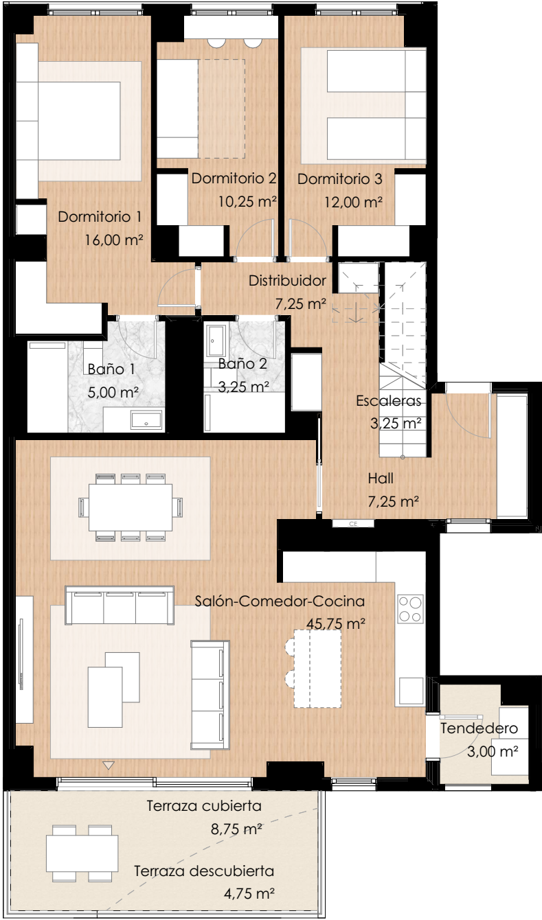
PLANTA 2
