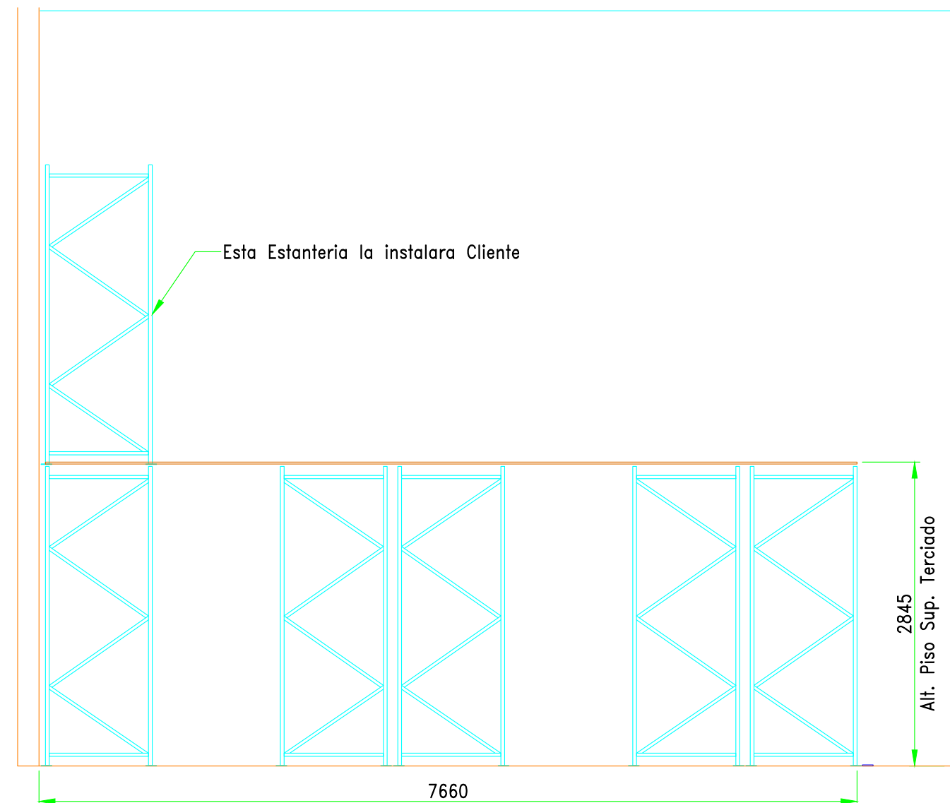
VISTA FRONTAL PLATAFORMA EXIST.
