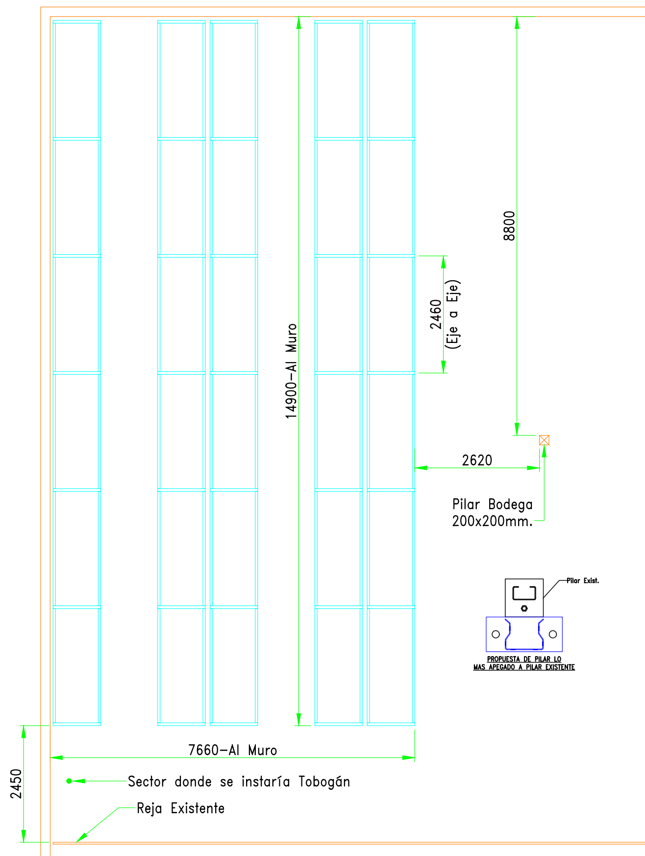
PLANTA DE ESTRUCTURAS EXISTENTES
