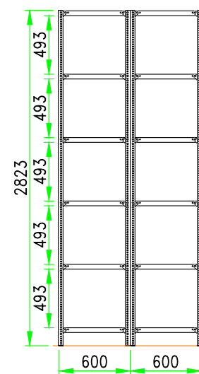
VISTA LATERAL EST. ANRA T.600
