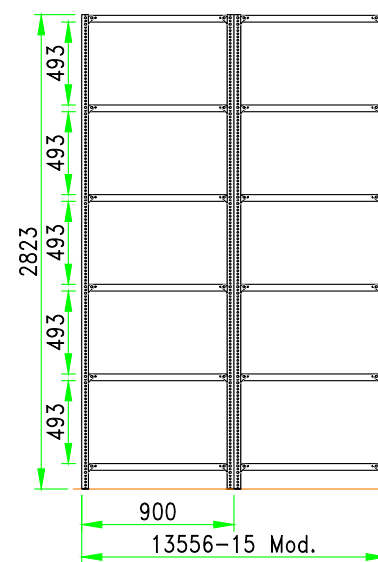
VISTA FRONTAL EST. ANRA
