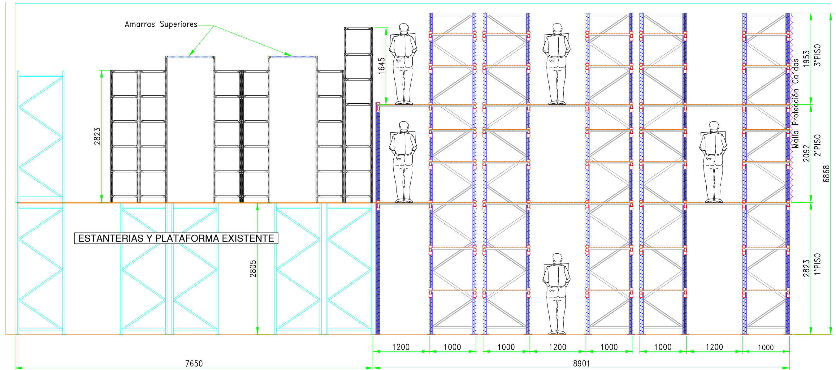
VISTA TRANSVERSAL ESTANTERIAS 3 PISOS
