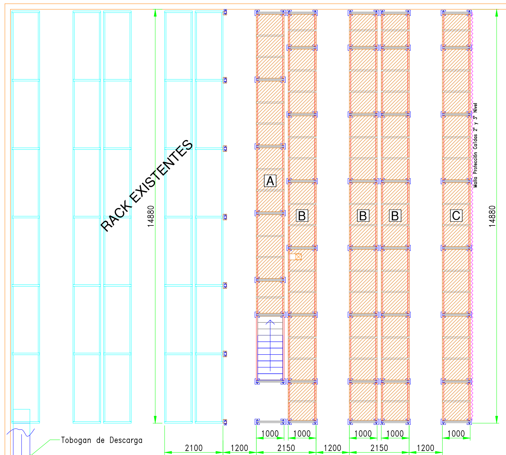
PLANTA DE DISTRIBUCION DE ESTANTERIAS 1° PISO
