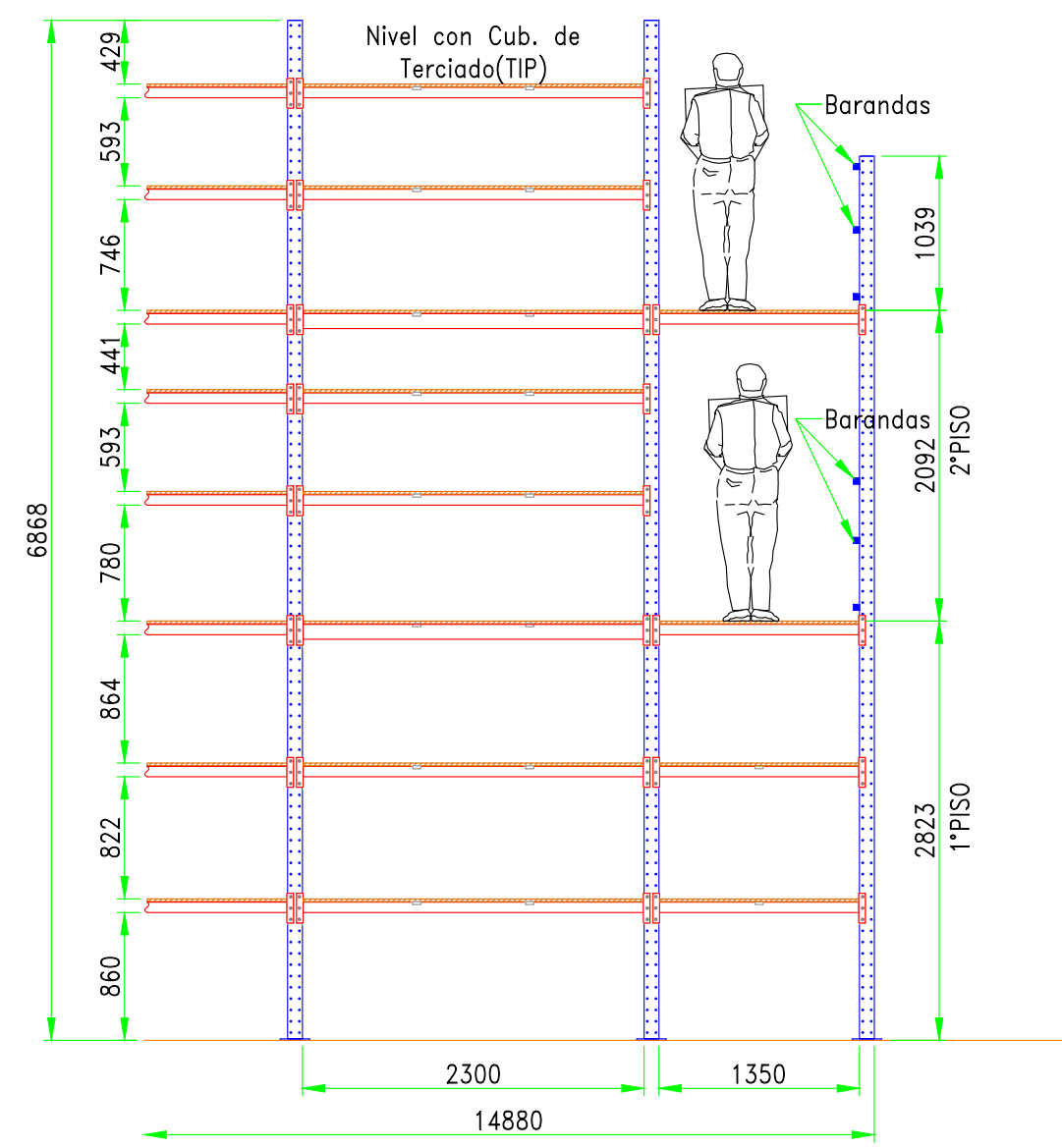
VISTA FRONTAL ESTANTERIAS 3 PISOS
